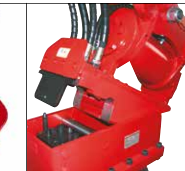
HUPPQuick-System: Hydraulikanlüsse werden beim Schnellwechselvorgang automatisch verbunden
